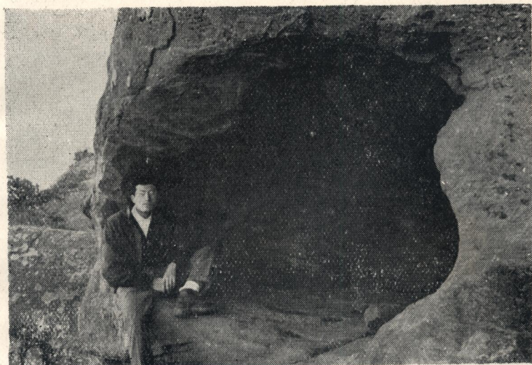
Bauma del Calamot. Puede apreciarse la estratificación cruzada de las areniscas, las cuales contienen algunos cantos de cuarzo y paleozoicos.
